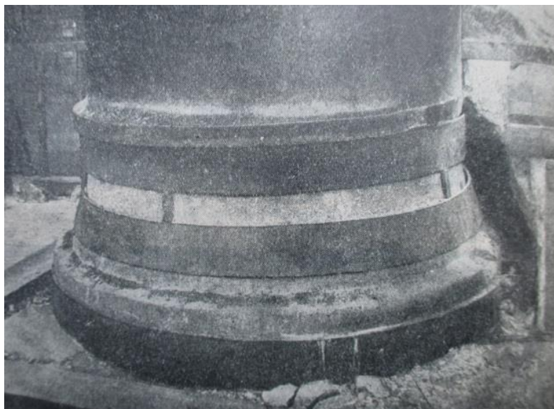
Рис. 5. Состояние оснований колонн портиков до и в процессе ремонтно-реставрационных работ под руководством Н.П. Никитина в 1927-1928 гг.
